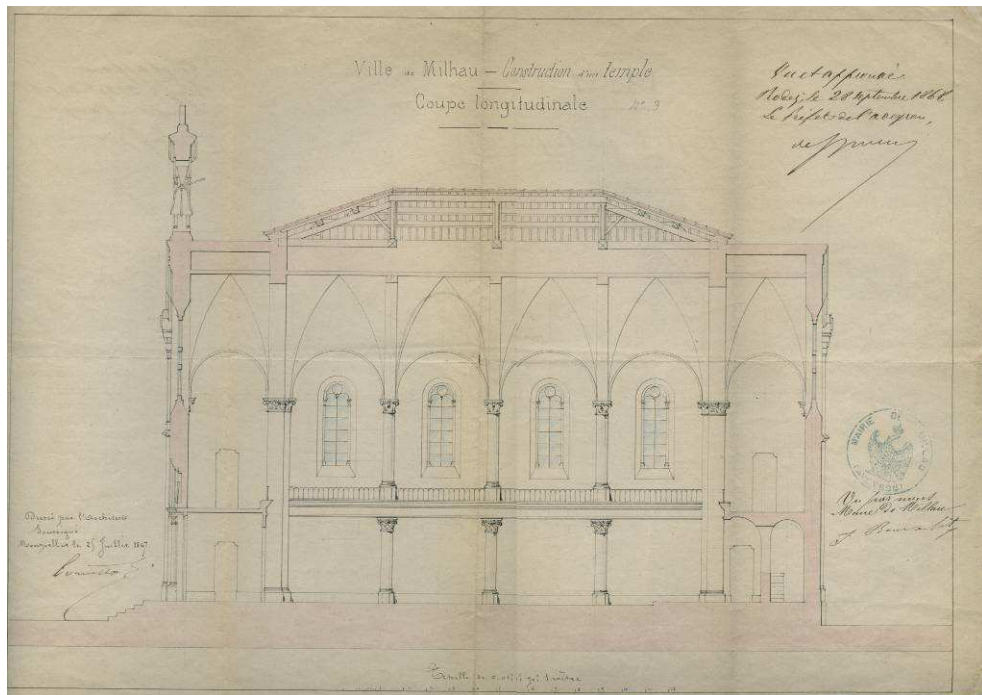
Coupe longitudinale du Temple par l'architecte Corvetto, de Montpellier (AMM).
